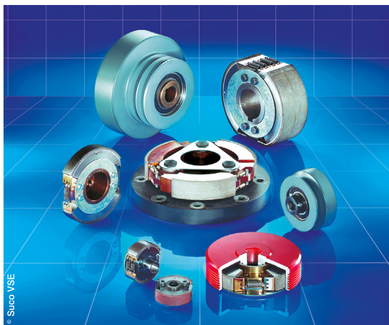
Embrayages/freins centrifuges Suco compacts et robustes, de 1 à 2000 N.m, poulie intégrée en option, versions personnalisées.
