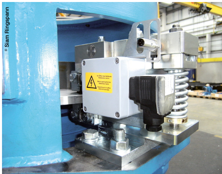
Frein électrique Siam Ringspann pour éolienne.
