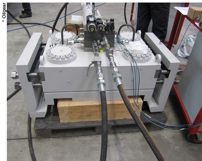
Bloc foré Oilgear monté sur vérin Douce Hydro.
