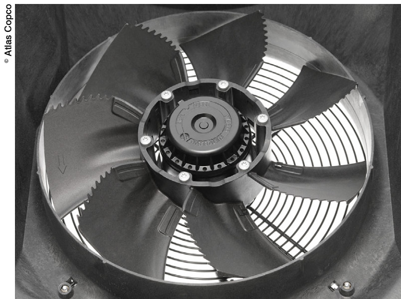
Conséquence du refroidissement par huile, de la meilleure efficacité du système de refroidissement air/huile et de l'absence de ventilateur en bout d'arbre, le niveau sonore est réduit de plusieurs décibels.
